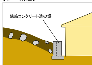
【塀の築造】
